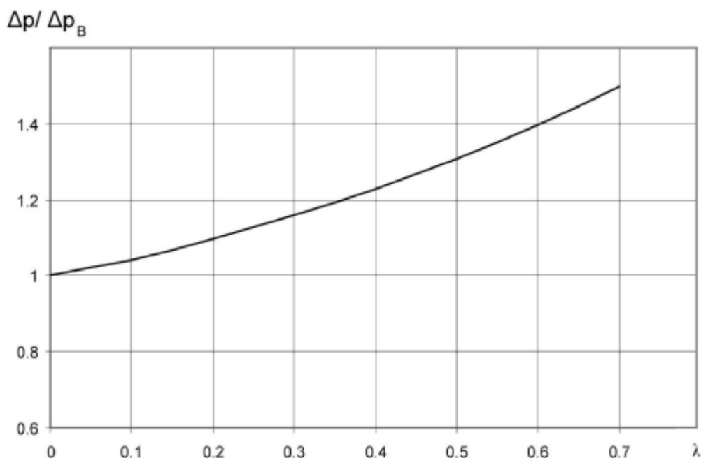
Рис. 1. Зависимость изменения относительного перепада давления \Delta p/\Delta p_B от величины коэффициента "сцепления" \lambda микрополярной жидкости; \Delta p – перепад давления в микрополярной жидкости, \Delta p_B – перепад давления из решения Бюргерса в ньютоновской жидкости.
