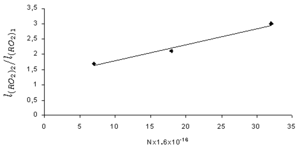
Рис. 2. Зависимость отношения величин сигналов ЭПР радикалов CH_3O_2 до (I_{RO_2})_1 и после (I_{RO_2})_2 реакции от количества поданного CH_4 .
