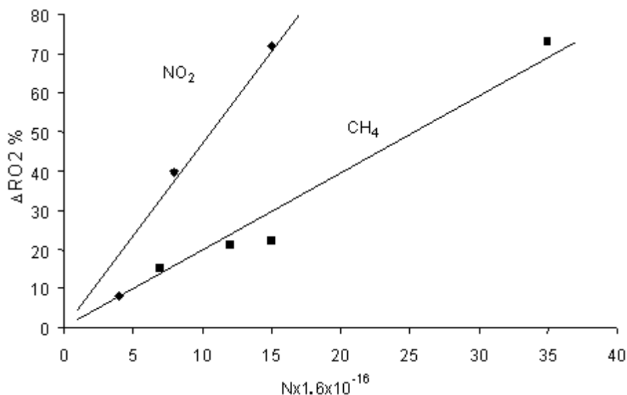
Рис. 1. Зависимость расхода радикалов \text{CH}_3\text{O}_2 от количества поданных \text{CH}_4 и \text{NO}_2 при T = 297 К.
